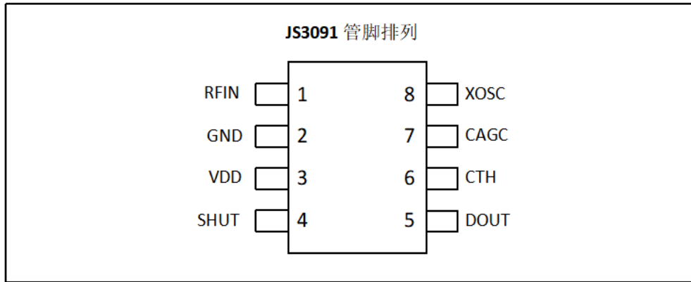
图 2 JS3091 管脚排列图
